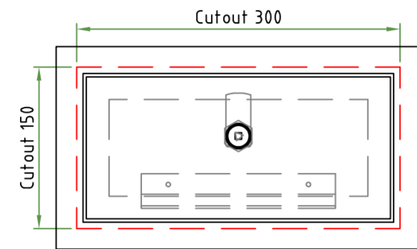
C-Steckklappe Drei-/Vierkant M 1:5
